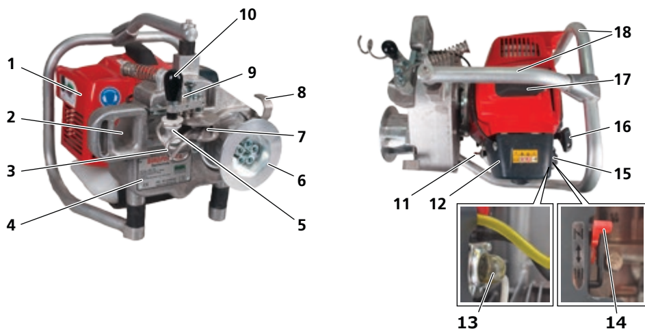
図 2 : カワサキエンジン搭載のキャプスタンウインチ1200
